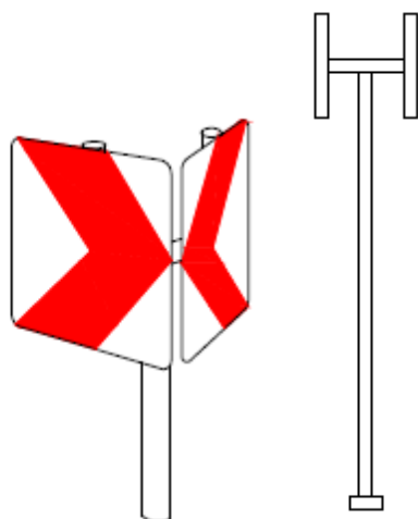
б) Разположение в хоризонтална крива на табели с направляваща стрелка C7
